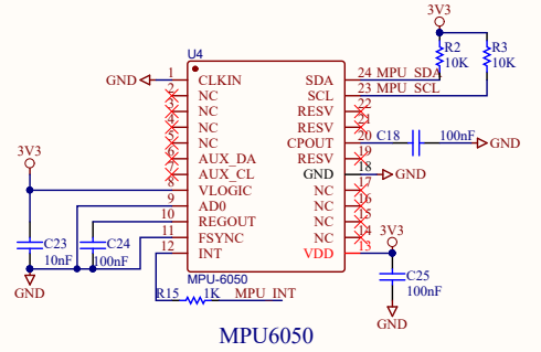
MPU6050
