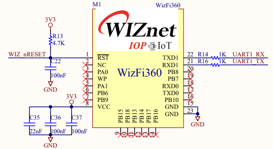
WizFi360
